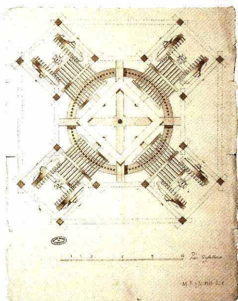
figura 7.- Planos del ingenio de Segovia
